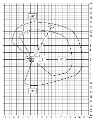
Abstützung einseitig – 50%
