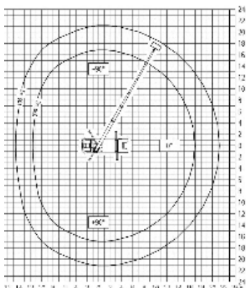
Abstützung beidseitig
