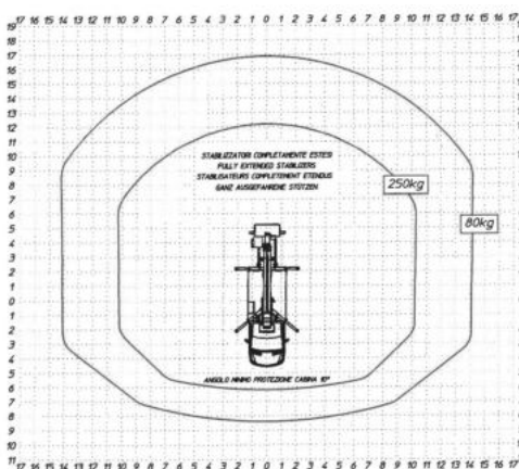
Abstützung beidseitig
